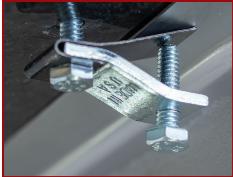
ACTUAL INSTALLATION
